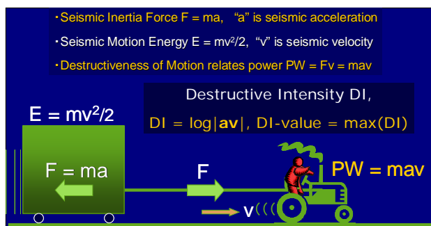
Fig.5 Definition of DI
