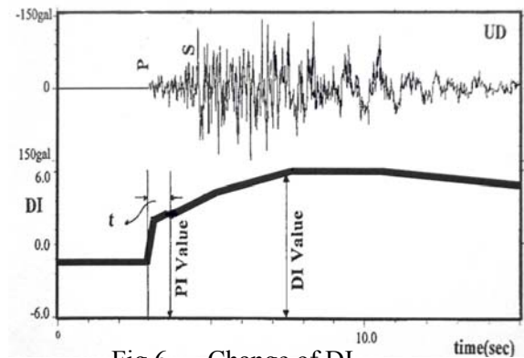
Fig.6 Change of DI
